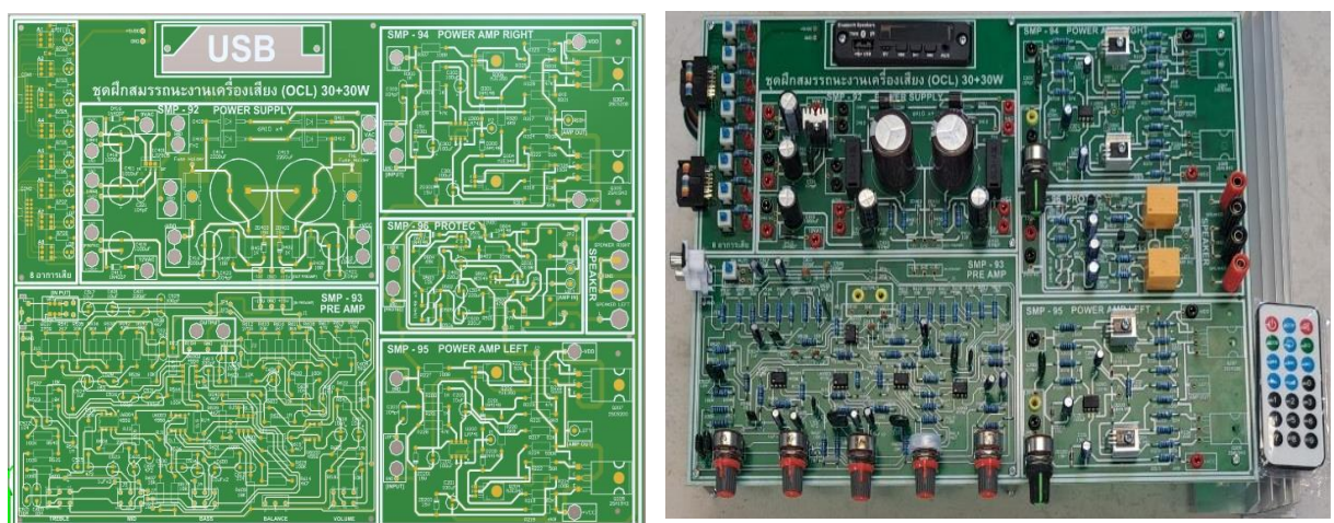
รูปที่ 4 แผ่น PCB และการวางอุปกรณ์ชุดฝึกสมรรถนะงานเครื่องเสียง SMP 92-96
