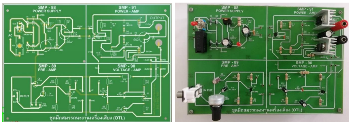
รูปที่ 3 แผ่น PCB และการวางอุปกรณ์ชุดฝึกสมรรถนะงานเครื่องเสียง SMP 88-91
